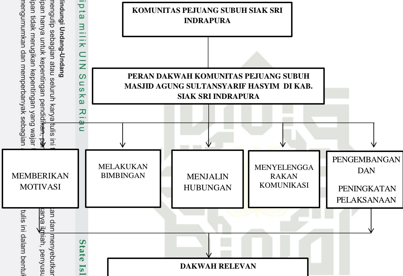
Gambar 4.1 Kerangka Pikir
