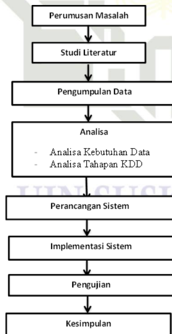
Gambar 1. Tahapan Penelitian
