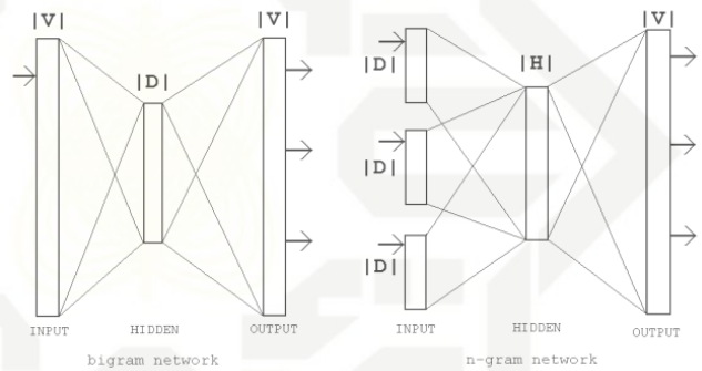
Gambar 2. Arsitektur dasar word2vec [17]
