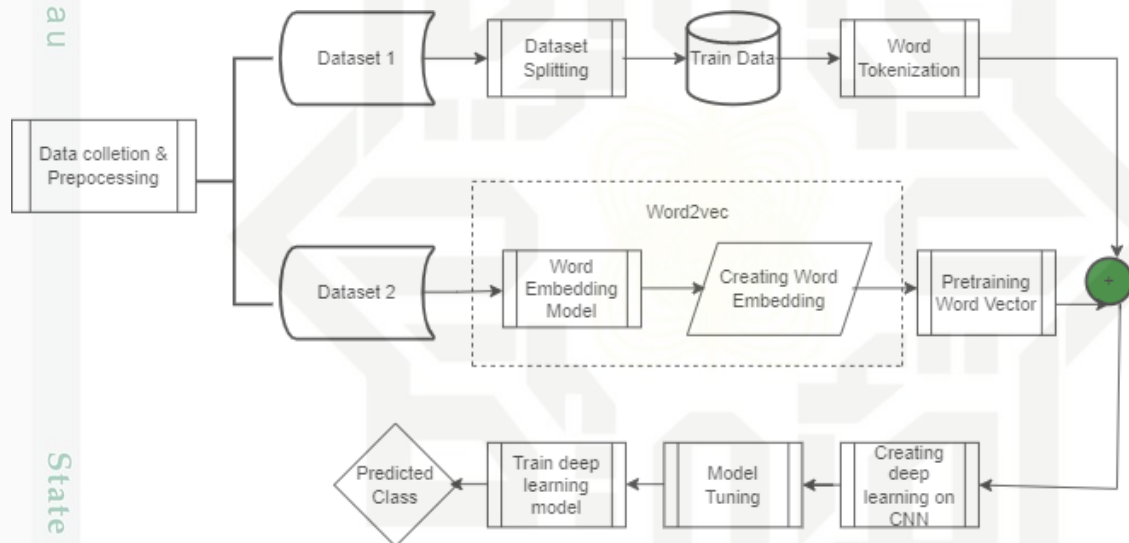
Gambar 5 Blok Diagram Tahapan Klasifikasi Tweet
