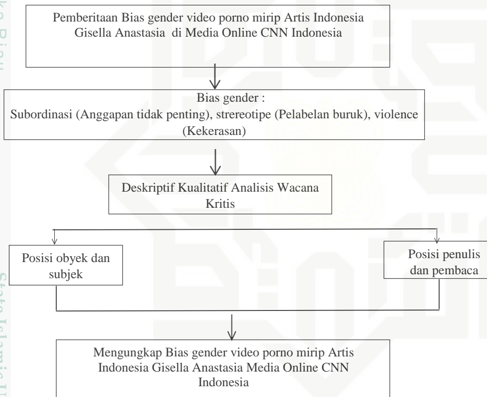
Gambar 2.1 Kerangka Berpikir
