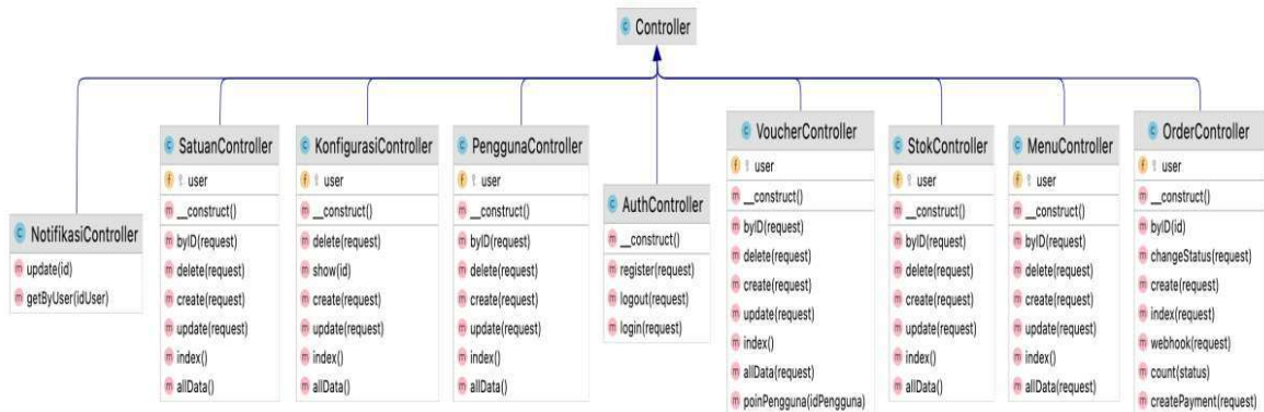
Gambar 4. 20 Class Diagram Aplikasi Reservasi Restoran Ikan Kopek Ndak Batulang Berbasis Mobile
