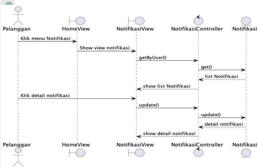
Gambar 4. 19 Sequence Diagram Melihat Notifikasi Pesanan
