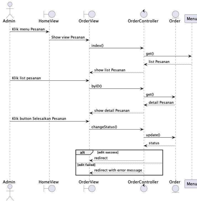
Gambar 4. 15 Sequence Diagram Mengelola Data Pesanan
