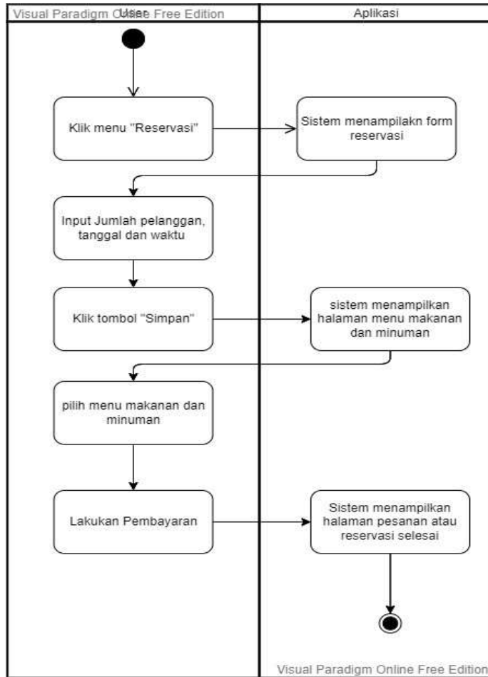
Gambar 4. 8 Activity Diagram Membuat dan Melihat Pesanan
