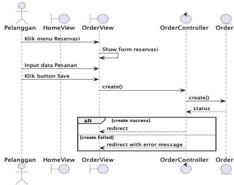
Gambar 4. 17 Sequence Diagram Membuat dan Melihat Pesanan
