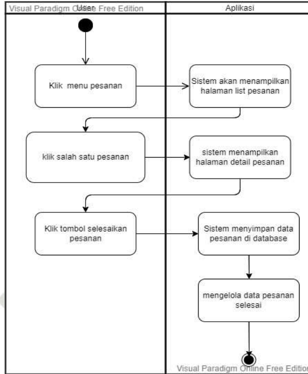
Gambar 4. 6 Activity Diagram Mengelola Data Pesanan
