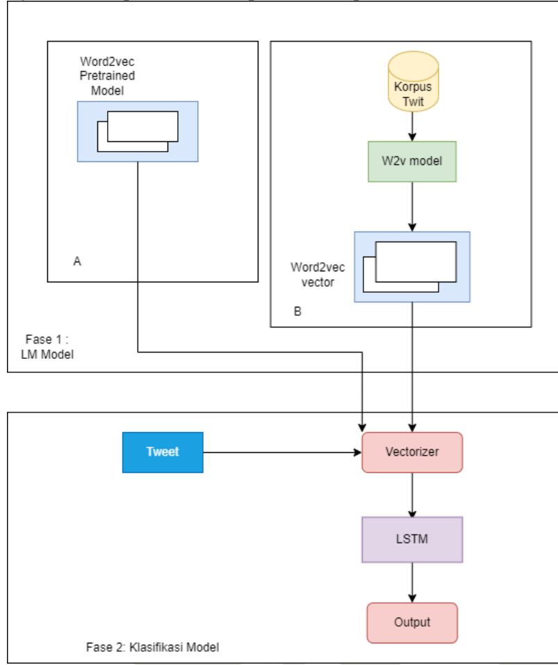
Gambar 3 Proses Klasifikasi dengan model word embeddings
