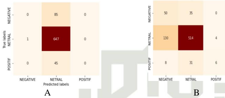
Gambar 7. Akurasi (dalam confusion matrix) terhadap pengujian data validasi (A) menggunakan data latih awal (B) menggunakan balanced train dataset
