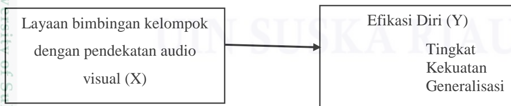
Gambar II. 1 Kerangka berpikir
