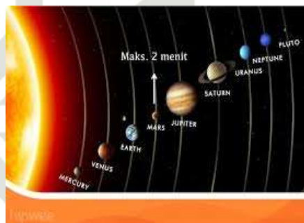
Gambar 2. 3 Planet-planet
