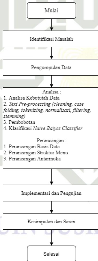
Gambar 1 Metodologi Penelitian
