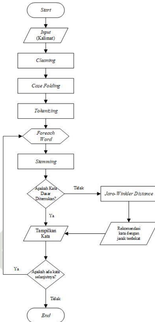
Gambar 3.2 Flowchart Analisa Normalisasi Teks
