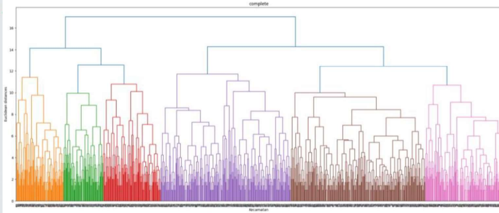
Gambar E.3 Dendogram metode Complete Linkage tahun 2017
