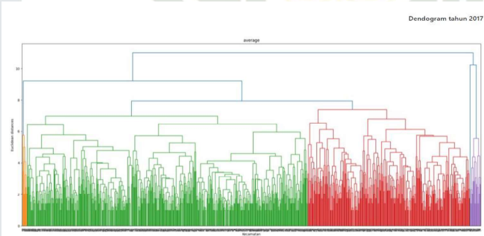
Gambar E.2 Dendogram metode Average Linkage tahun 2017
