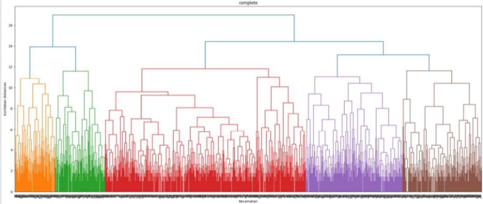
Gambar E.9 Dendrogram metode Complete Linkage tahun 2019
