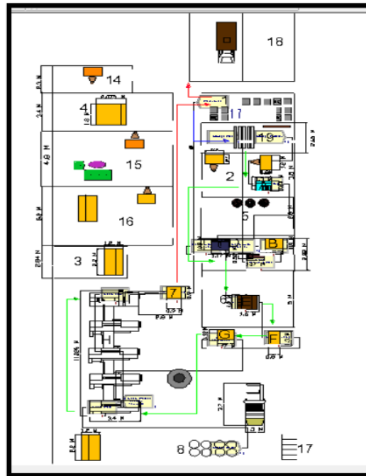
Gambar 10 Simulasi Layout Usulan
