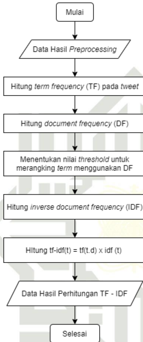
Gambar 4. 8 Flowchart Ekstraksi Fitur TF - IDF
