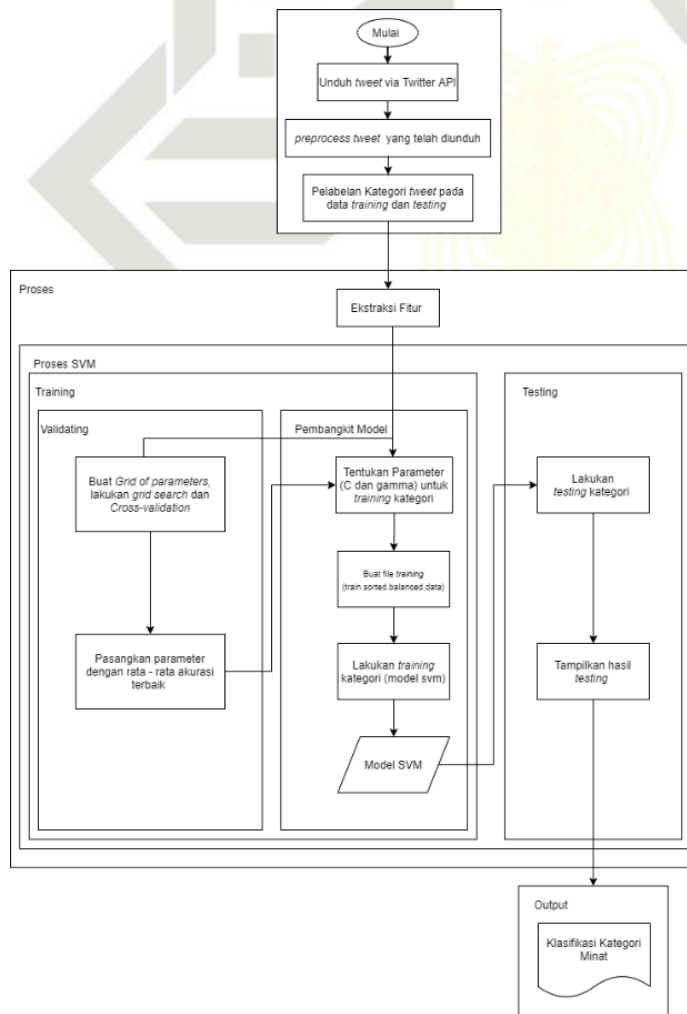
Gambar 4. 5 Deskripsi Umum Secara Keseluruhan
