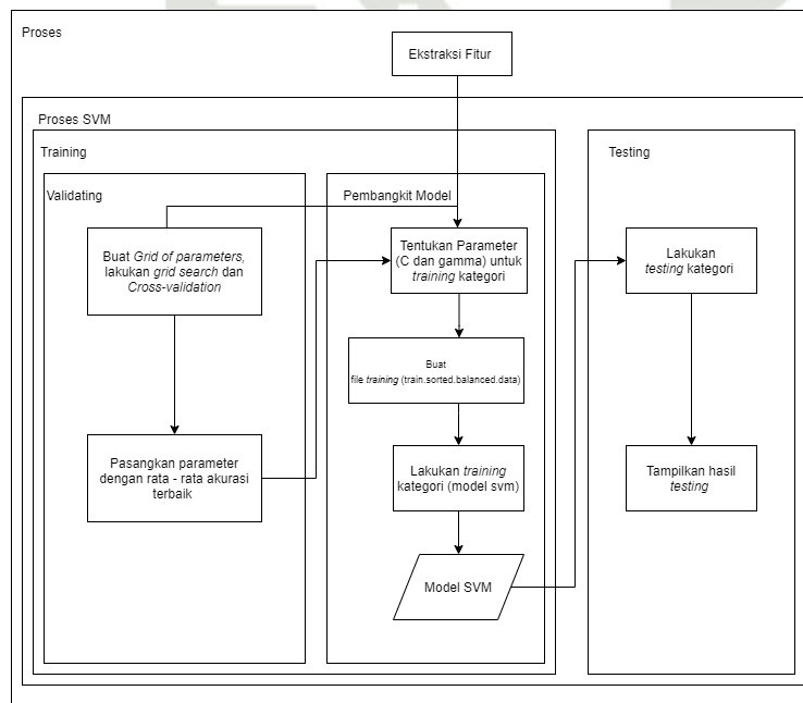
Gambar 4. 3 Deskripsi Umum (Proses)
