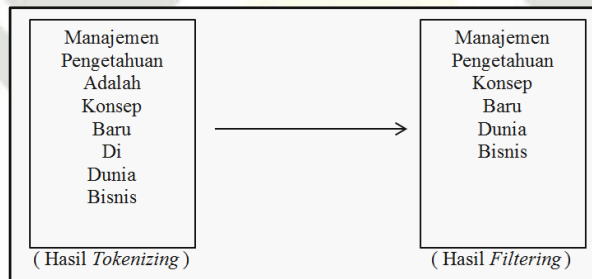
Gambar 3.3 Tahapan Filtering
