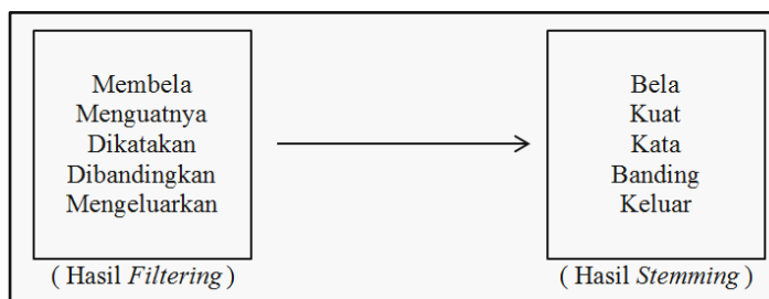
Gambar 3.4 Tahapan Stemming
