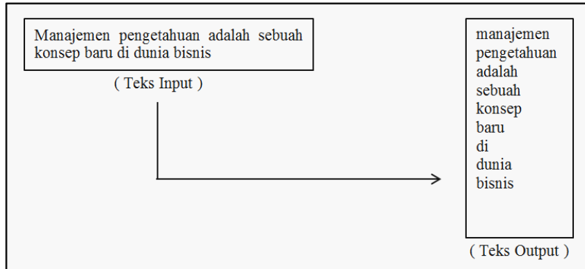
Gambar 3.2 Tahapan Tokenizing
