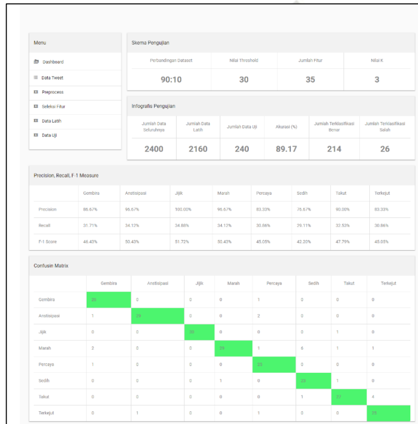
Gambar 5.7 Implementasi Antarmuka Halaman Pengujian
