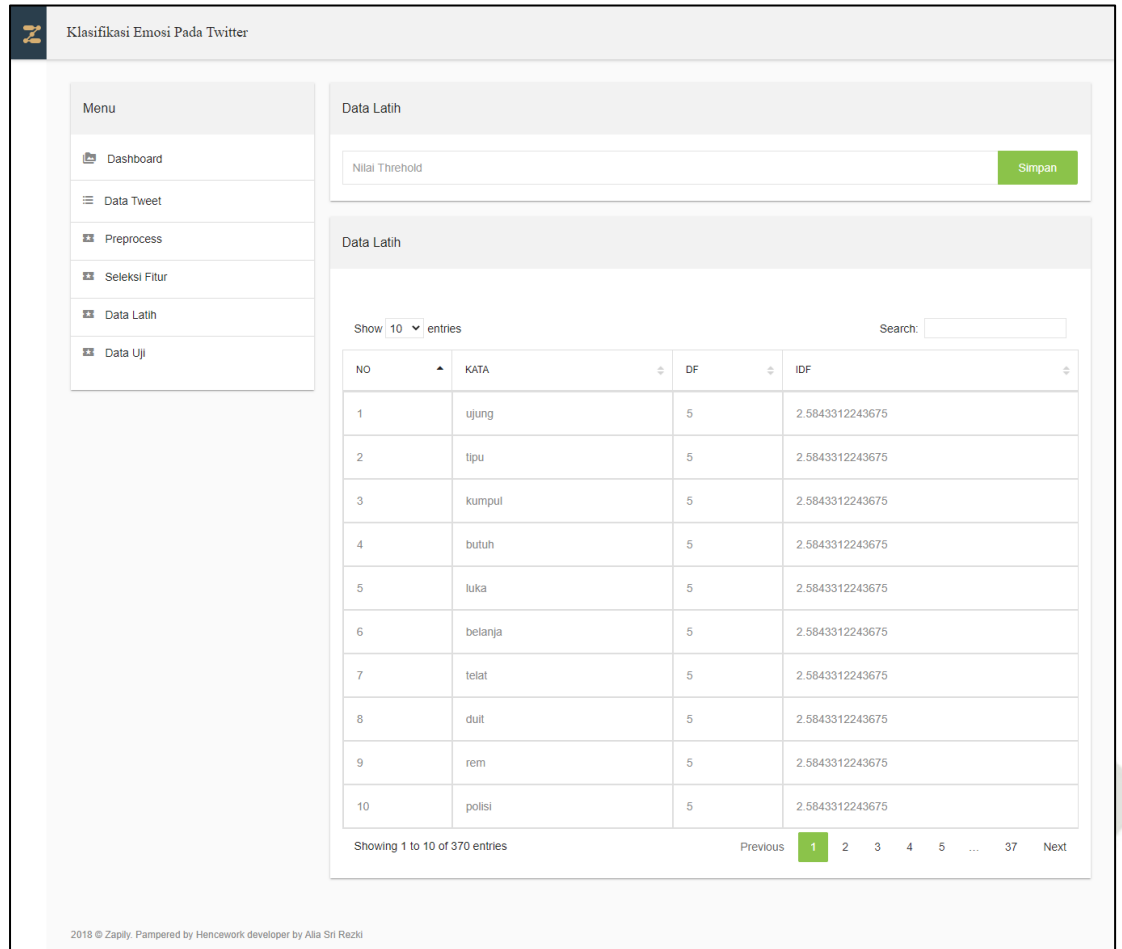
Gambar 5.4 Implementasi Antarmuka Halaman Seleksi Fitur
