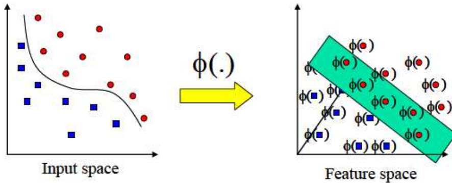
Gambar 2.6 Perpindahan Dari Vektor Input Ke Feature Space
