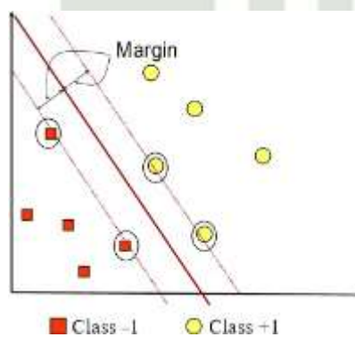
Gambar 2.5 Konsep Hyperline Pada SVM
