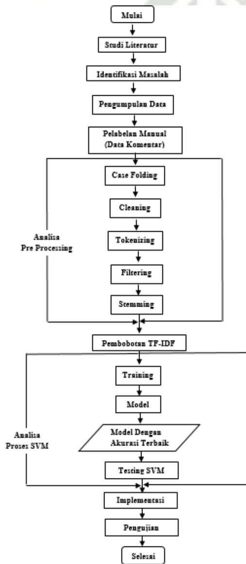
Gambar 3.2 Tahapan Penelitian
