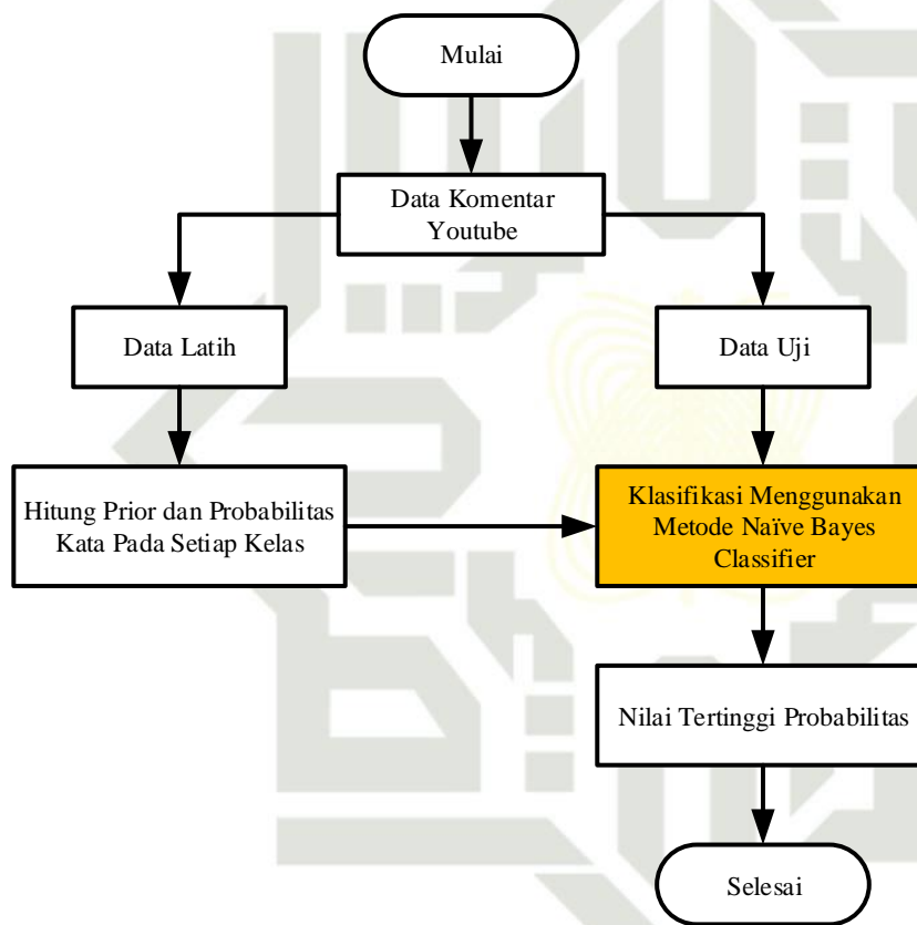
Gambar 4. 3 Flowchart Klasifikasi dengan Naïve Bayes Classifier
