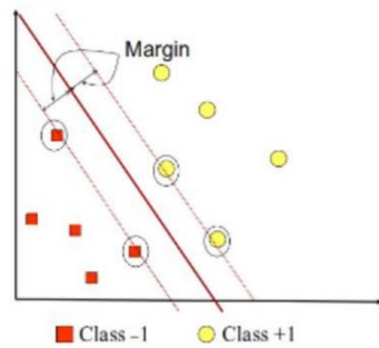
Gambar 2.1 Konsep Hyperplane pada SVM
