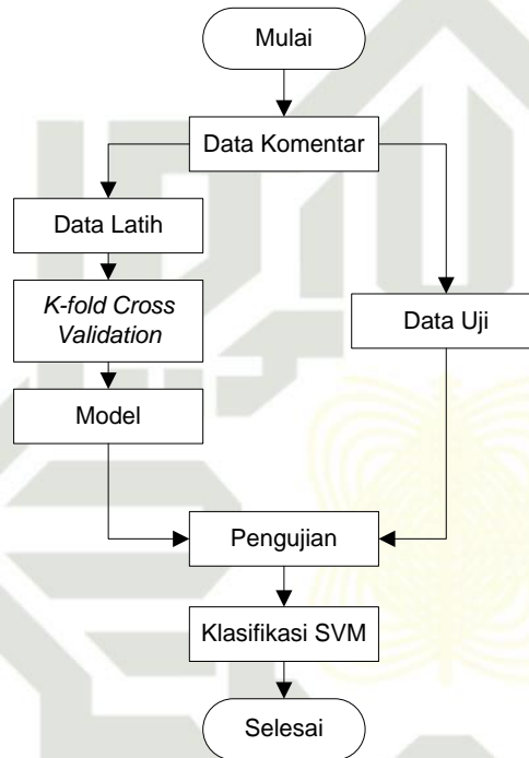
Gambar 3.2 Tahapan Metode SVM
