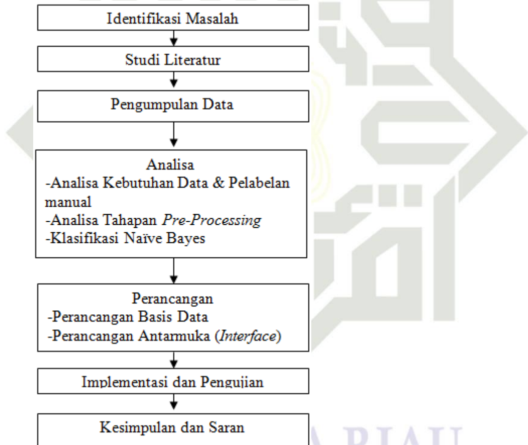
Gambar 3.1 Metodologi Penelitian
