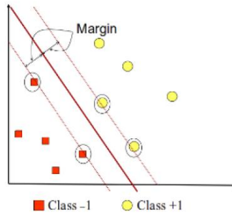
Gambar 2.1 Konsep Hyperplane pada SVM (Asiyah & Fithriasari, 2016)
