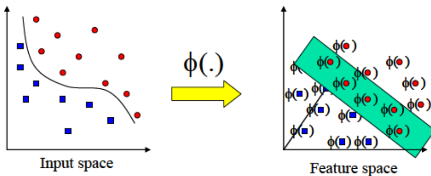
Gambar 2.2 perpindahan dari vektor input ke feature space (Sembiring, 2007)
