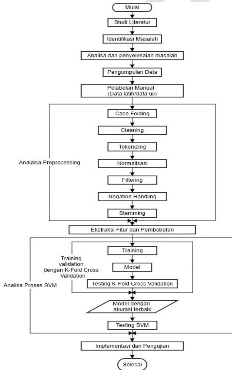
Gambar 3.1 Tahapan Penelitian
