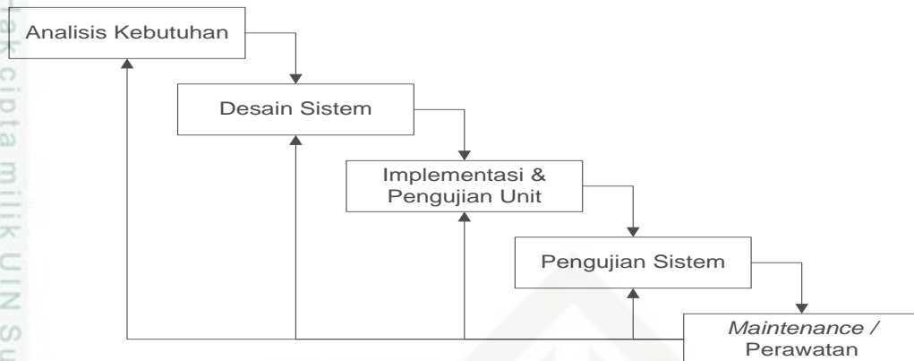
Gambar 2.4. Metodologi Waterfall
