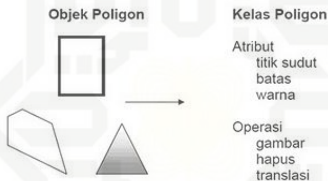
Gambar 2.3. Kelas dan Objek
