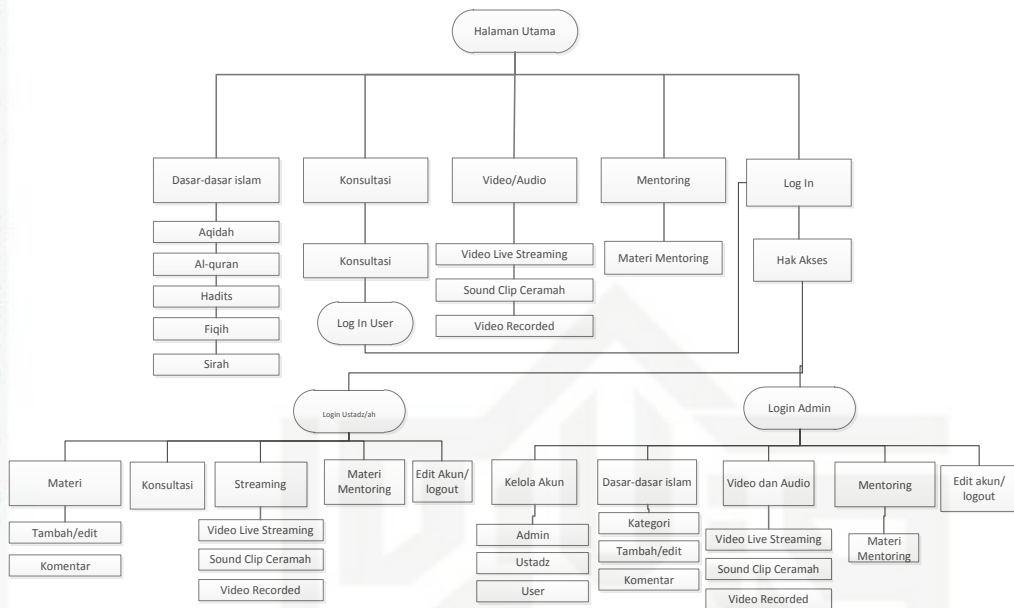
Gambar 4.34 Struktur Menu
