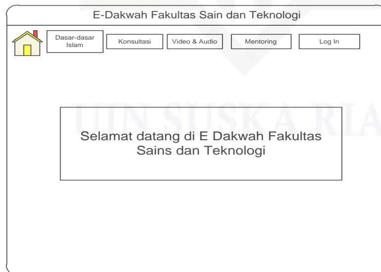
Gambar 4.36 Menu Utama
