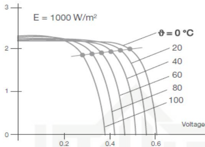
Gambar 2.9 Grafik Pengaruh temperatur modul pada produksi energi modul surya (Sumber Permadi 2008)
