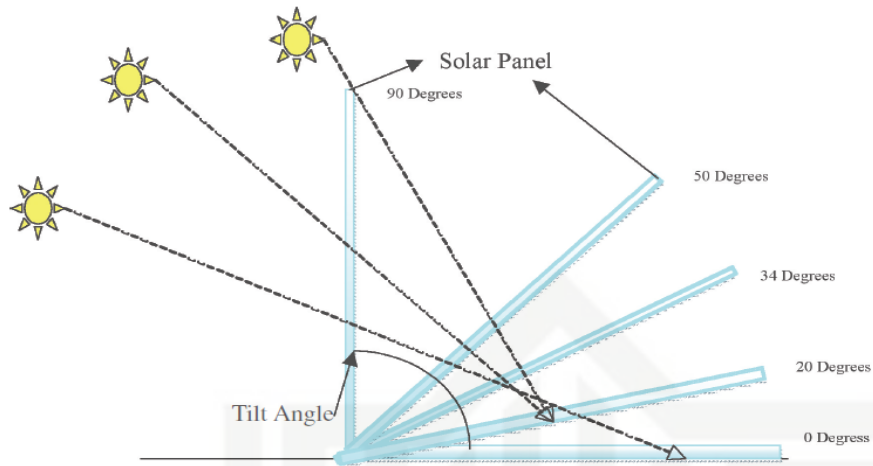
Gambar 2.12 Pemasangan PV Module dengan sudut kemiringan [18] (Sumber Alhamda 2015)
