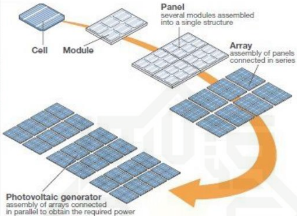
Gambar 2.8 Diagram Hubungan Antara Solar Cell , Modul , Panel dan Array (Sumber ABB 2010)
