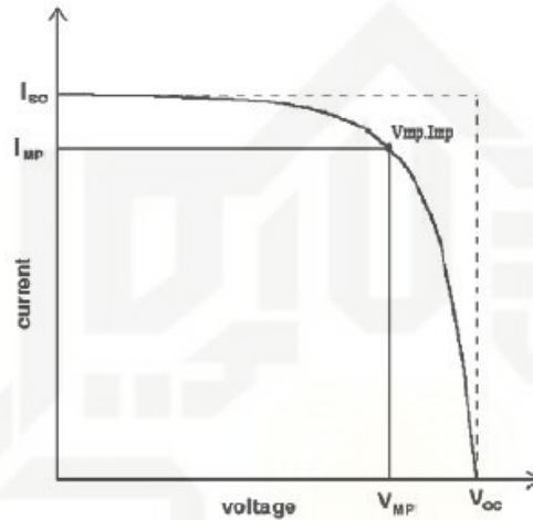
Gambar 2.7 Grafik Kurva I-V Pada Modul Sel Surya
