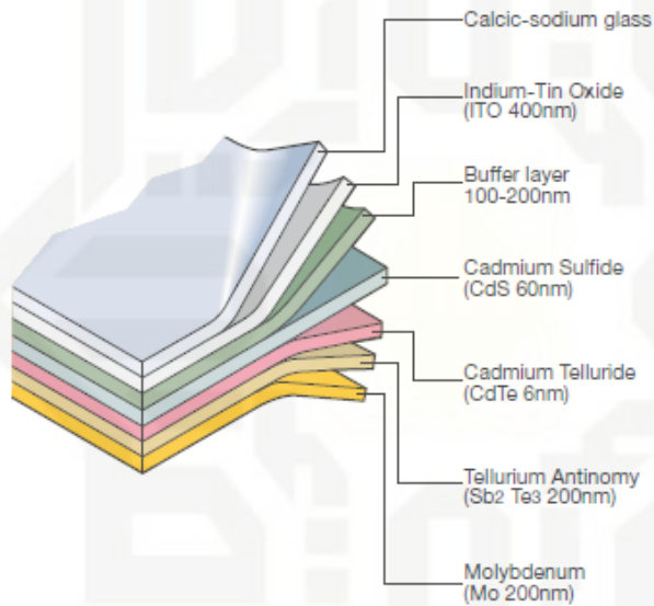
Gambar 2.6 Struktur Thin Film Dengan Bahan CdTe-CdS (Sumber ABB 2010)
