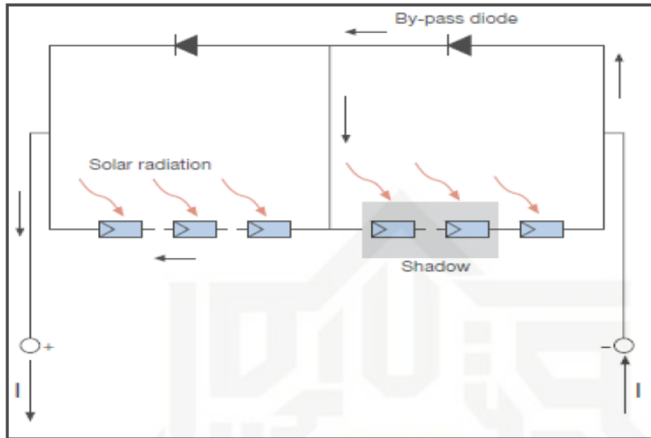
Gambar 2.10 Pengaruh Shading Terhadap Modul Surya (Sumber ABB 2010)
