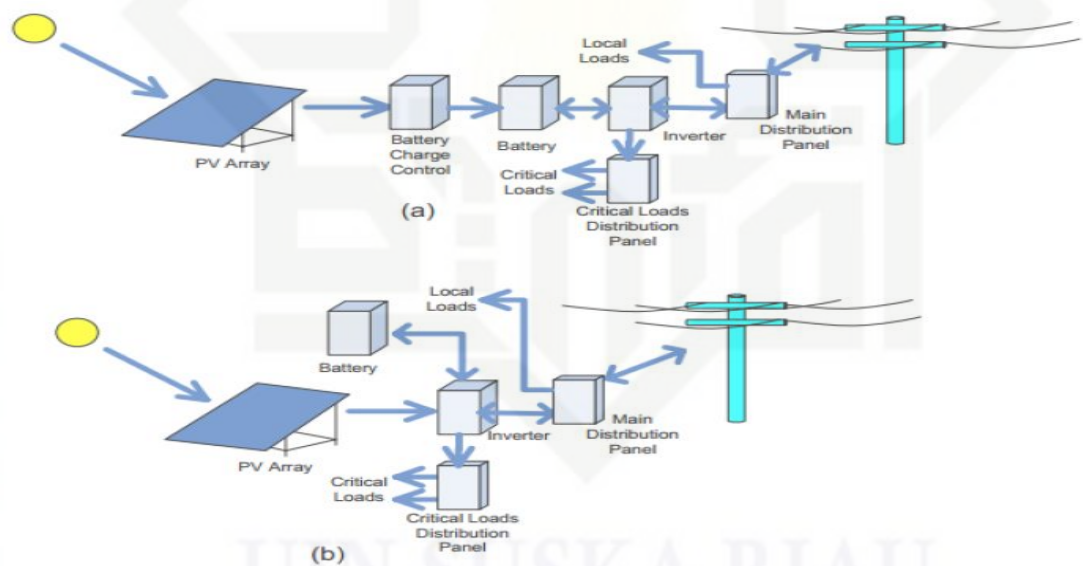
Gambar 2.1 Sistem PLTS grid-connected Dengan Penyimpanan ( Storage ) (a) Charge Control dan Inverter Charge Control Terpisah, dan (b) Charge Control Terintegrasi (Sumber ABB 2010)
